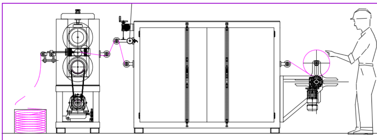
Avvolgitore per nastri
